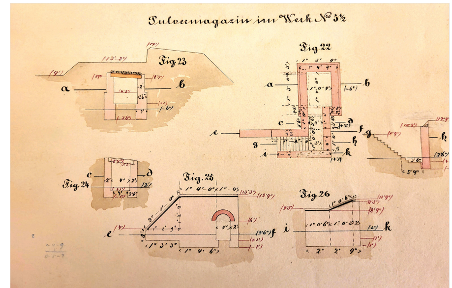
Detailplan eines Pulvermagazins
